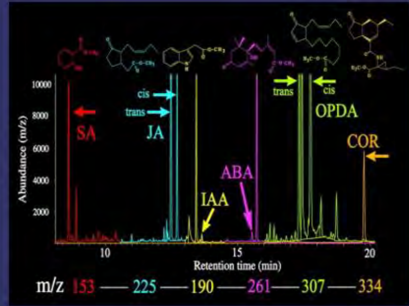
chromatogramma-spettro MS
